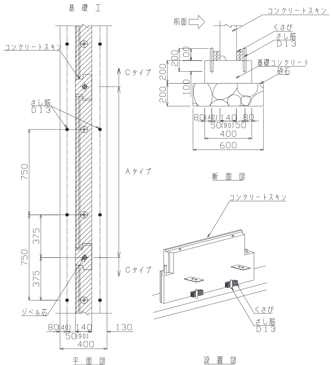
圖-23 基礎工断面図
