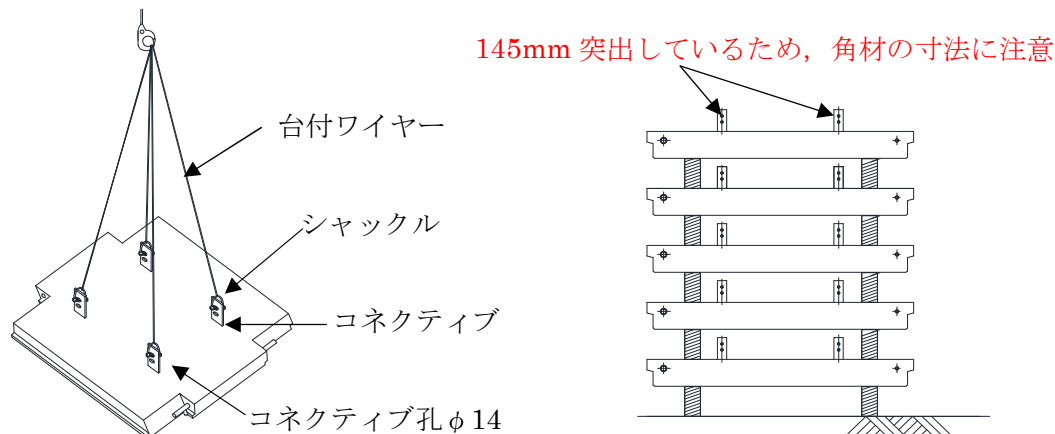
図-21 コンクリートスキン
