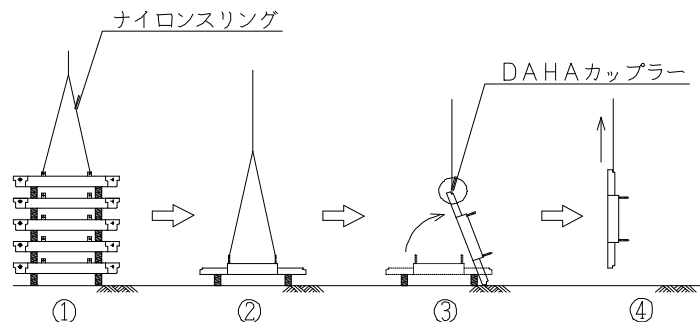
図－３０ 吊り上げ手順
