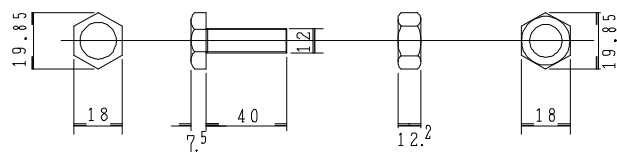
図－１６ ボルト・ナット
