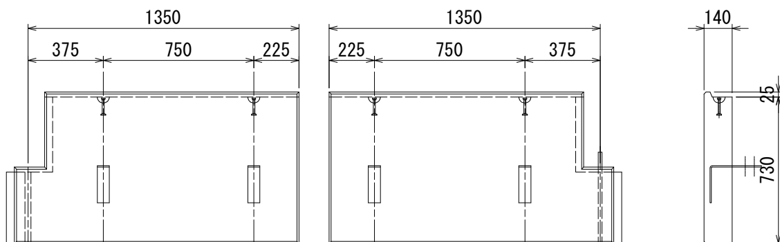
図－ 1 0 端部加工タイプ・最下段用 (CR 2, CL 2)
