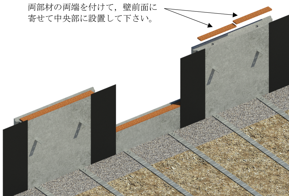
図-36 水平目地材の設置方法
