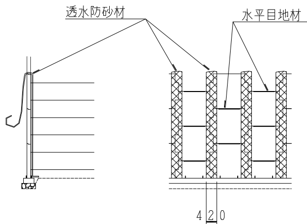
図-35 透水防砂材の敷設方法
