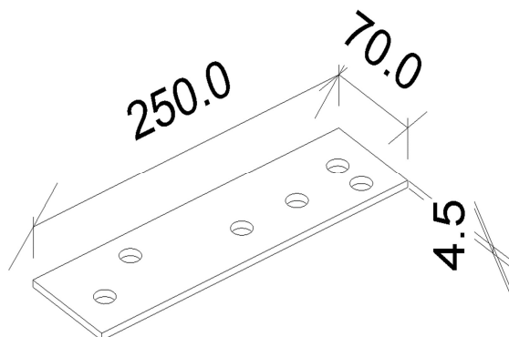
図-19 ガセットプレート (Nタイプ)
