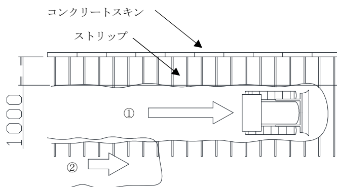
図-39 大型機械の走行
