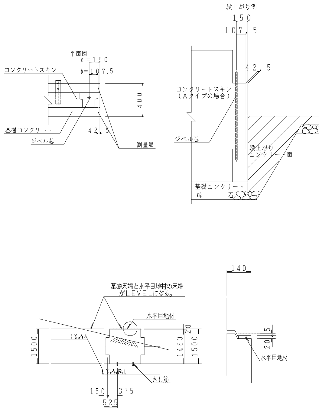
図－２４ 段上り部
