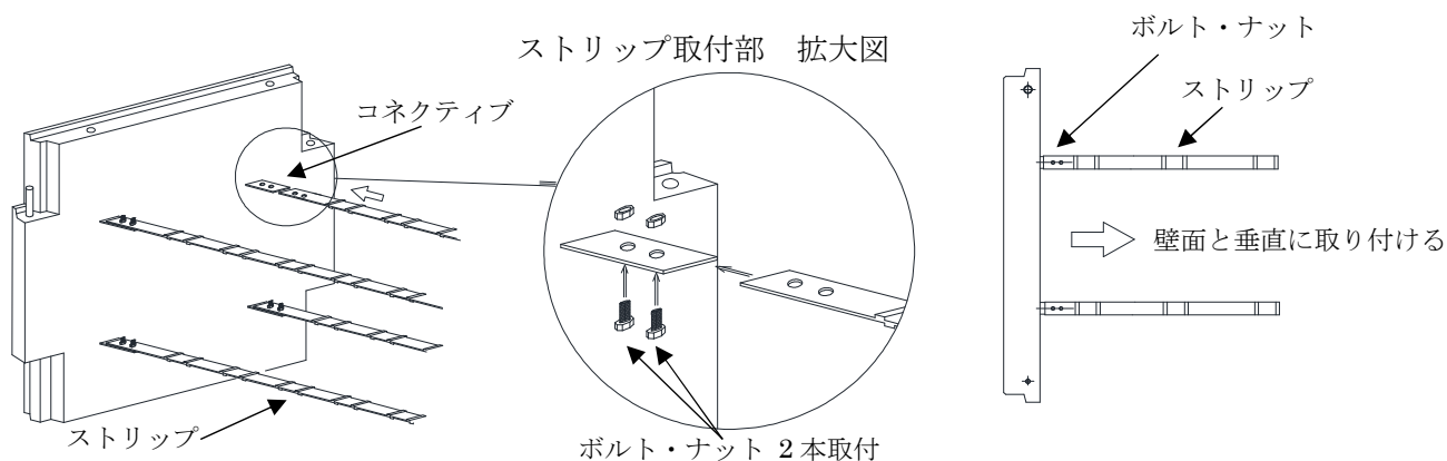
図-25 スキンパネルの組み立て
