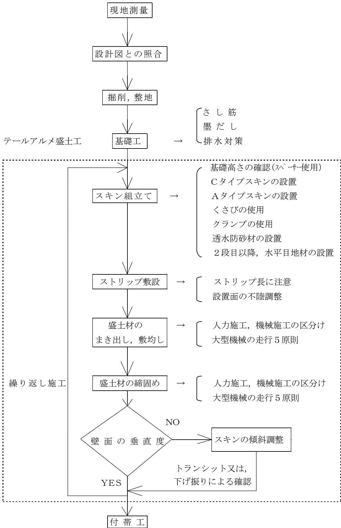
図-20 施工手順
