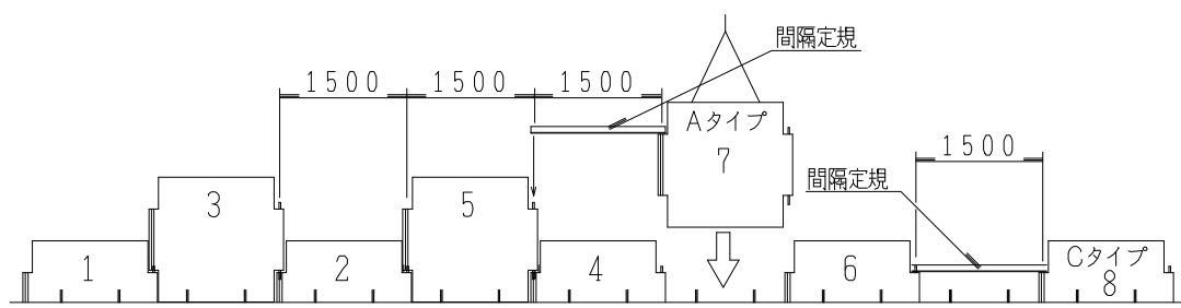
図-25 スキンパネルの組み立て
