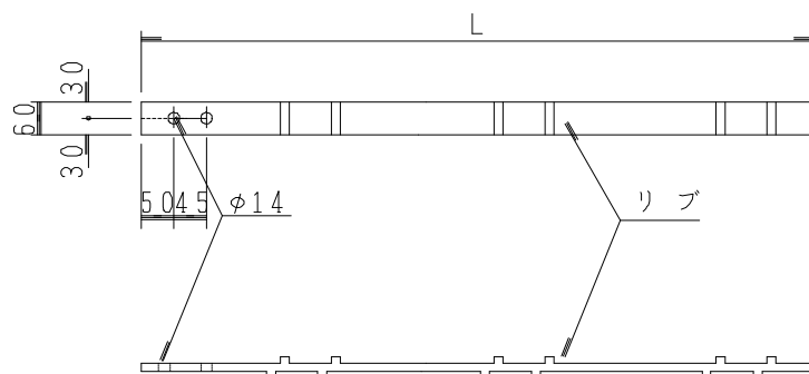
図-14 ストリップ
