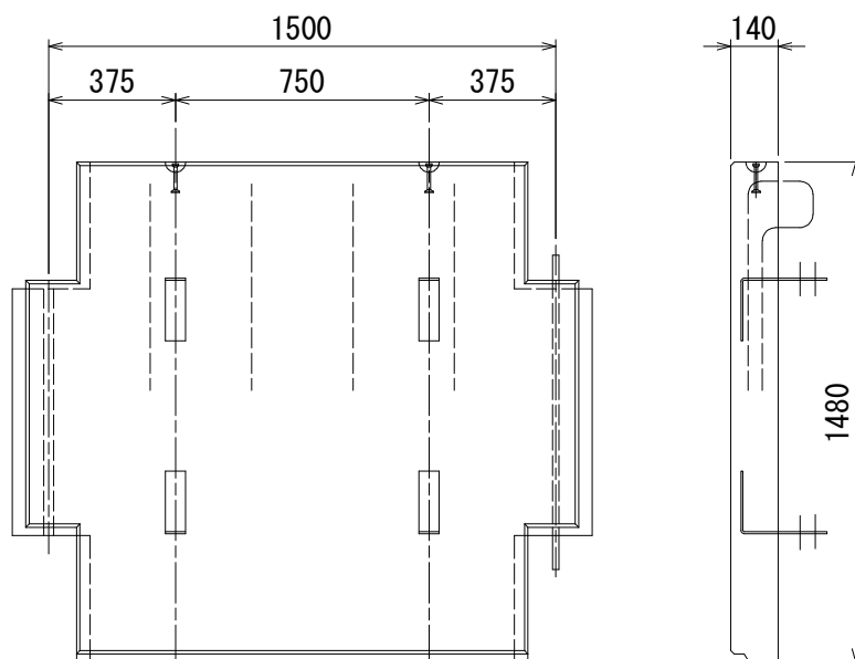
図－6 天端用タイプ (BP4)
