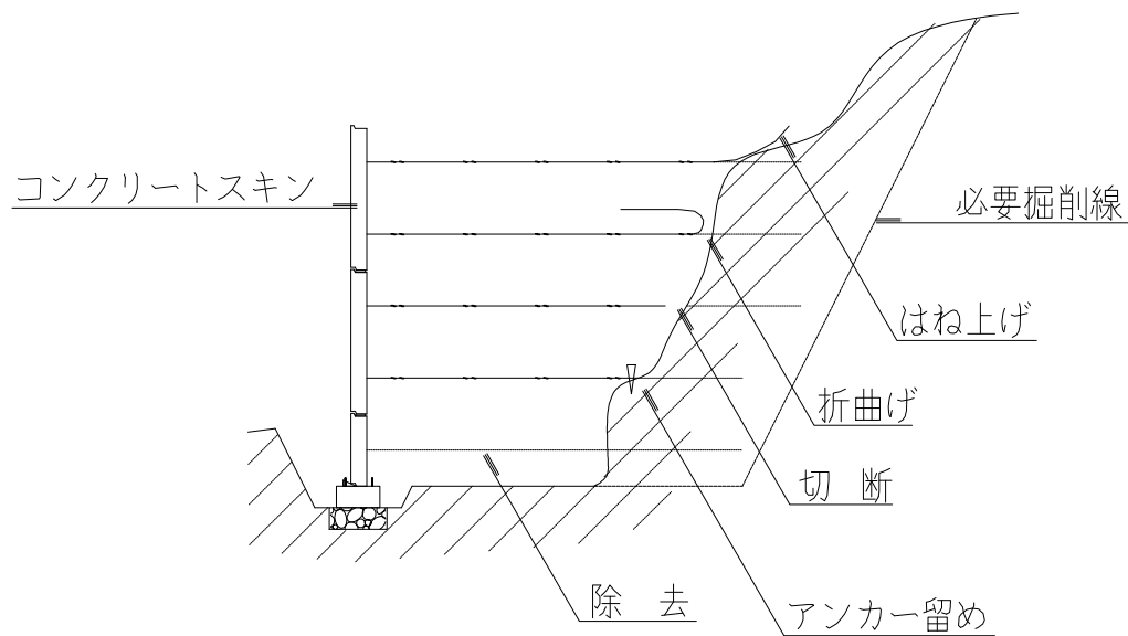
図-40 ストリップ取り付け時の禁止事項
