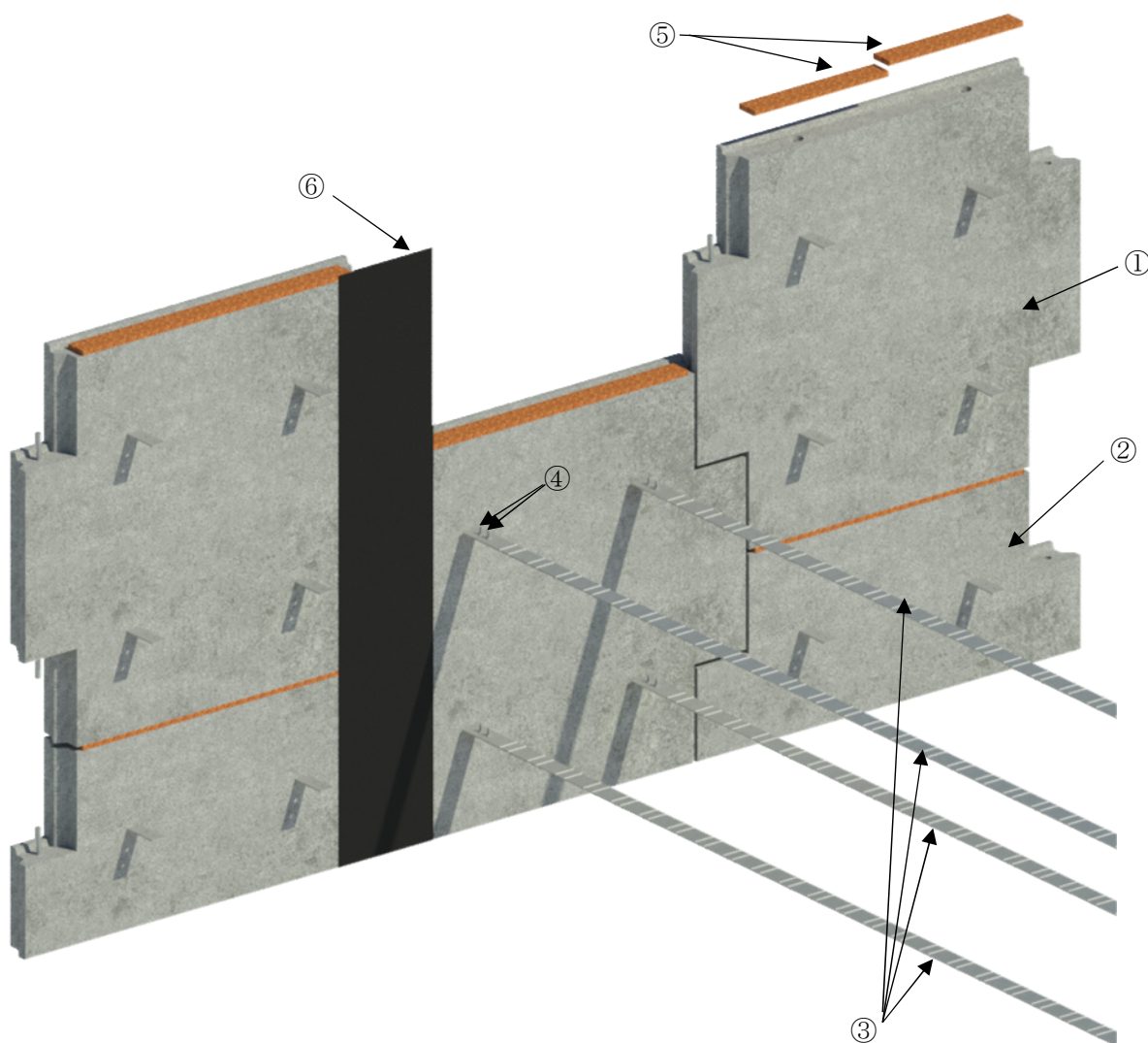
図－３ 構造図（裏面）
