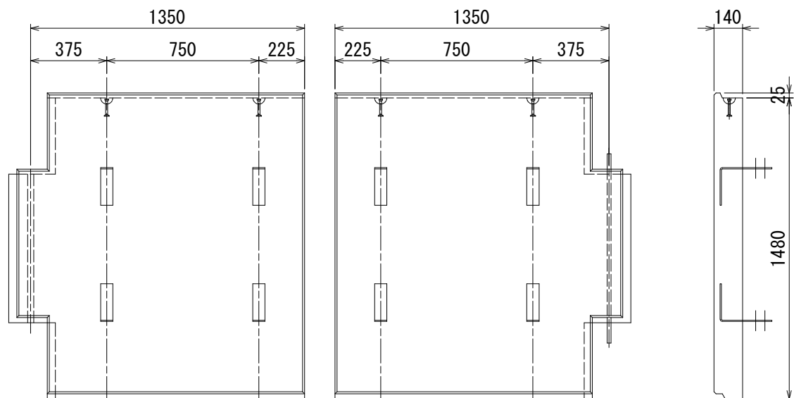
図－ 9 端部加工タイプ (AR 4, AL 4)
