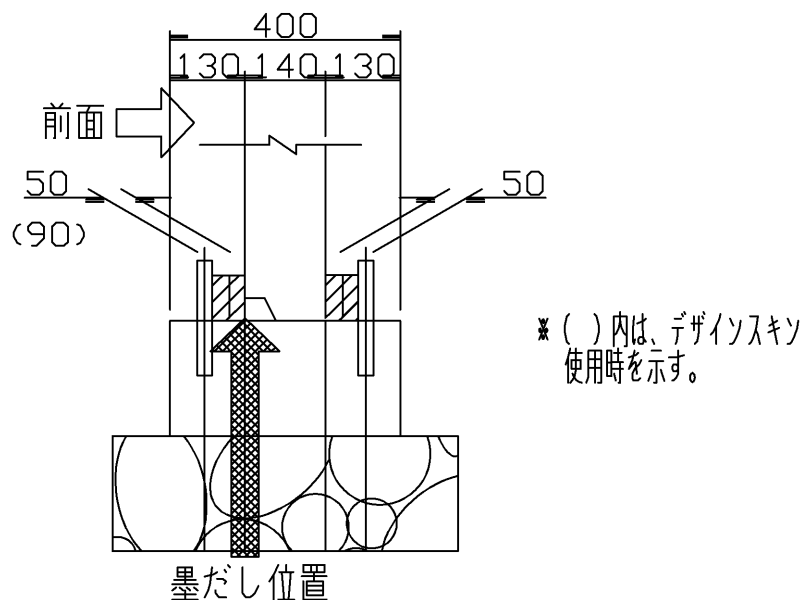
図－２８ 墨だし位置
