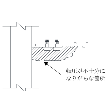
図-38 ストリップ取付図
