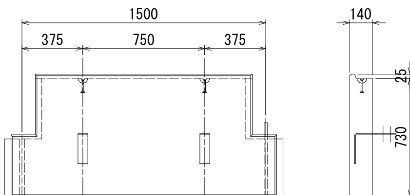
図－6 天端用タイプ (BP4)
