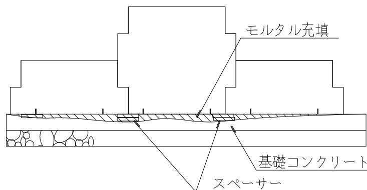
図－２９ スペーサーの使い方
