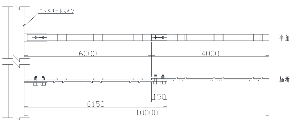
図-15 ストリップの連結例 ( L = 10 \text{ m} の場合)
