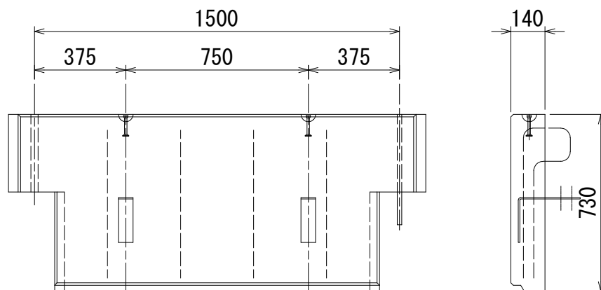
図－7 最下段用タイプ (C2)
