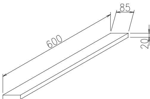
図－１７ 水平目地材
