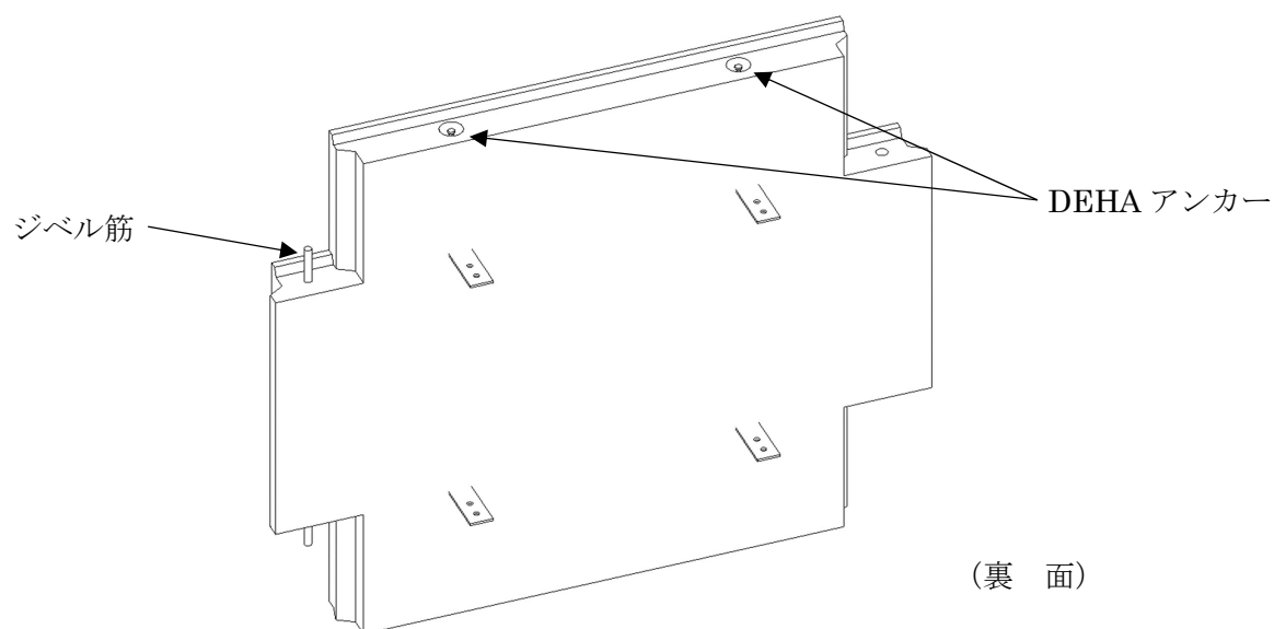
図-4 スキン構造図
