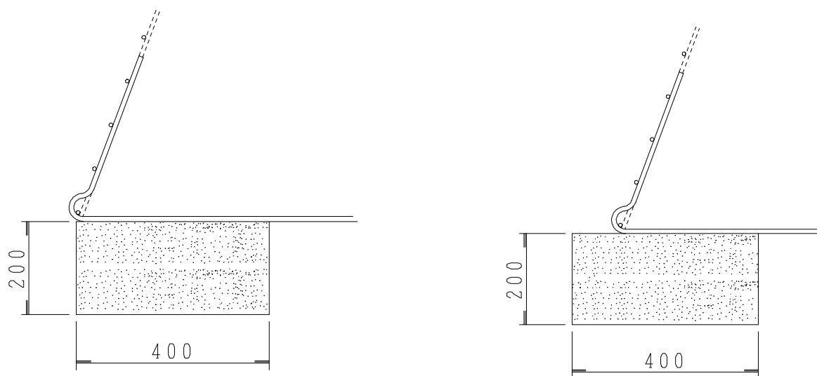
図－１１ 基礎工詳細図
