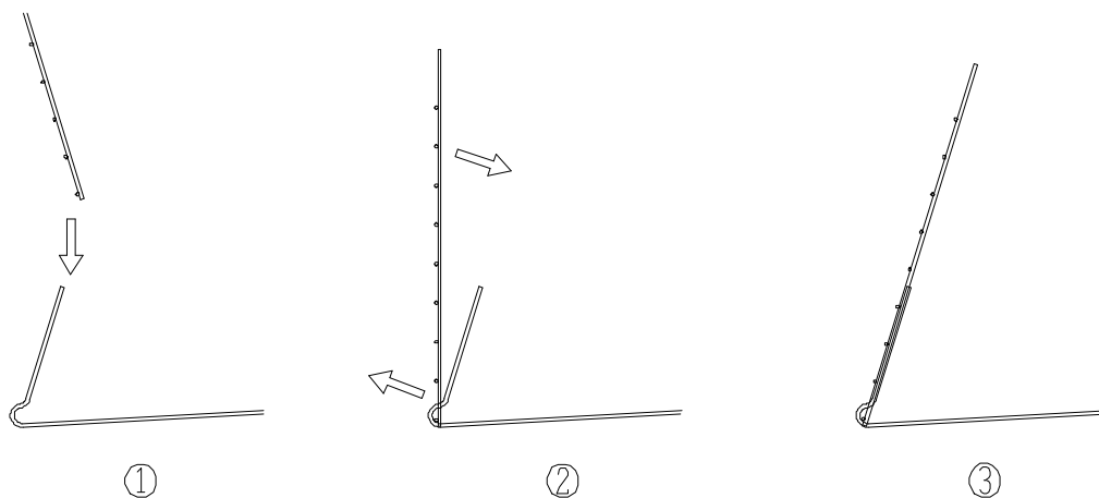
図－20 設置手順
