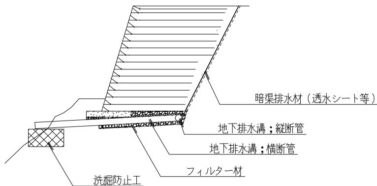
図-24 排水工例
