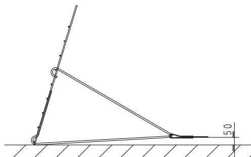
図－21 ストリップの敷設
