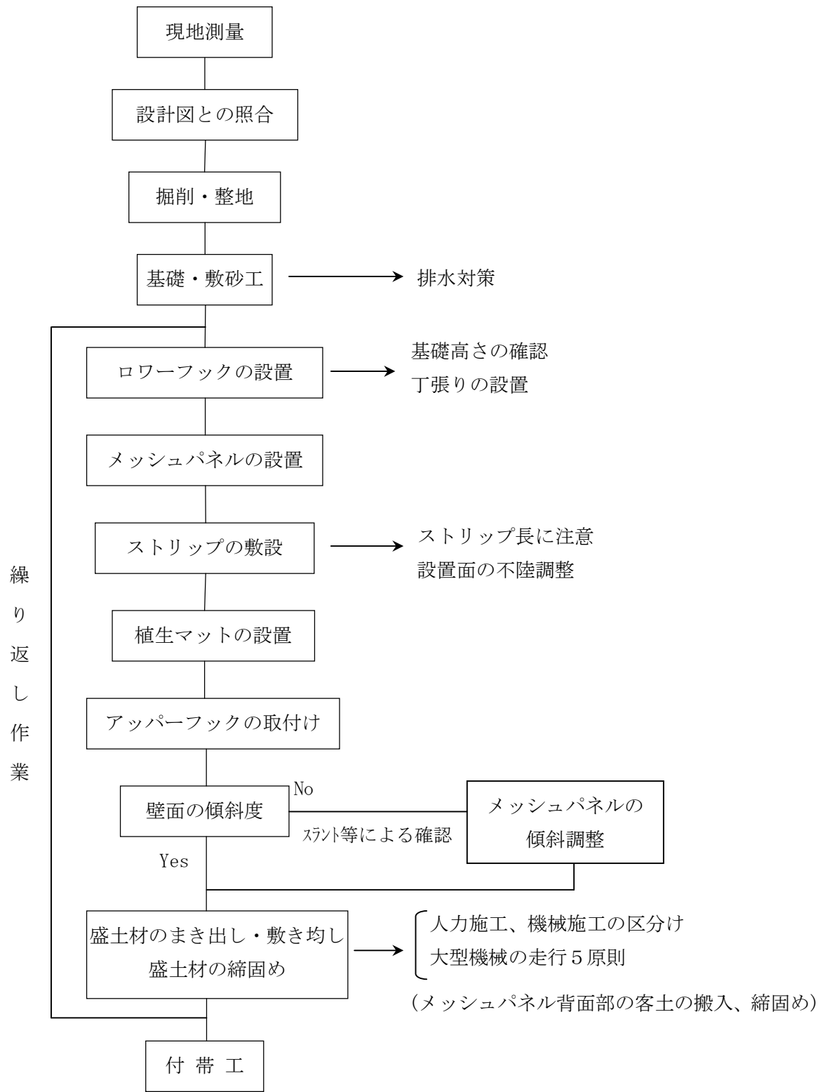
図－8 施工手順
