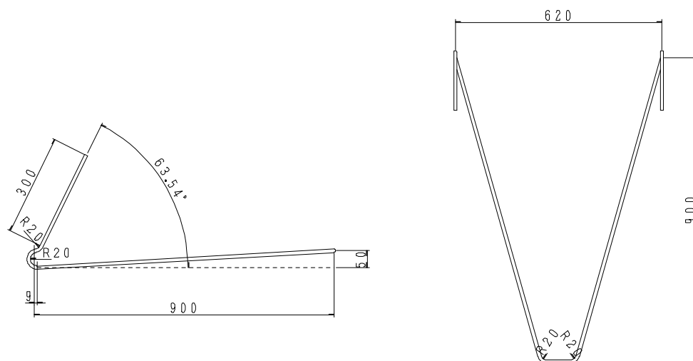
図－3 ロワーフック
