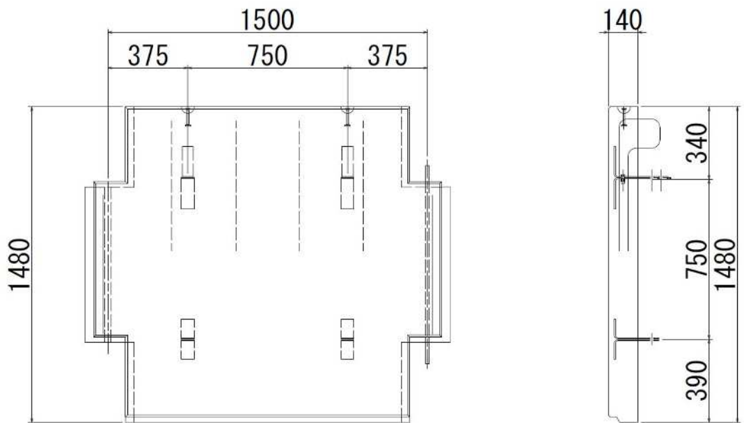
図-7 天端用タイプ ( F B P 4 )
