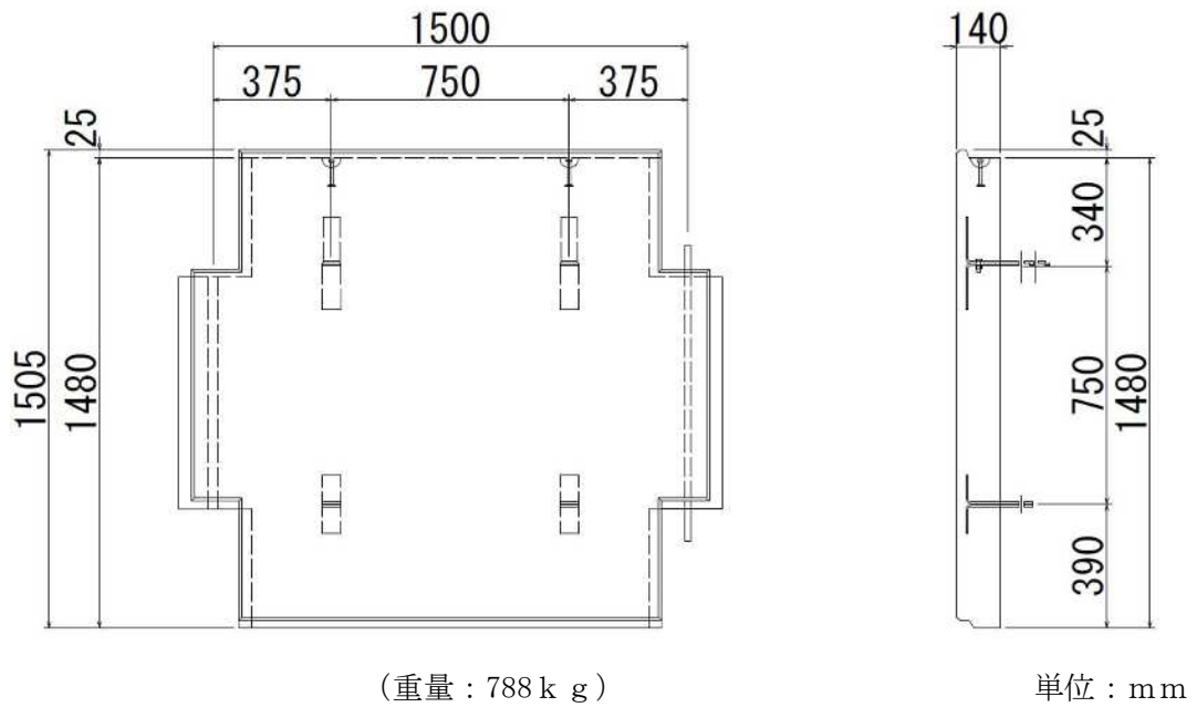
図-5 標準タイプ (FA4)
