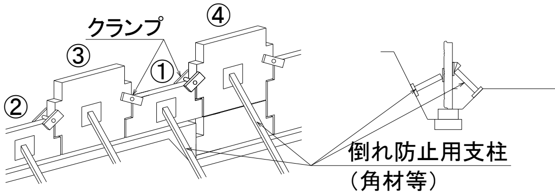
図-50 段上がり部の不安定なスキンとその固定方法の例
