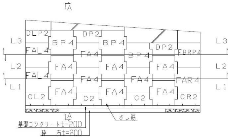
図-1 正面展開図 例
