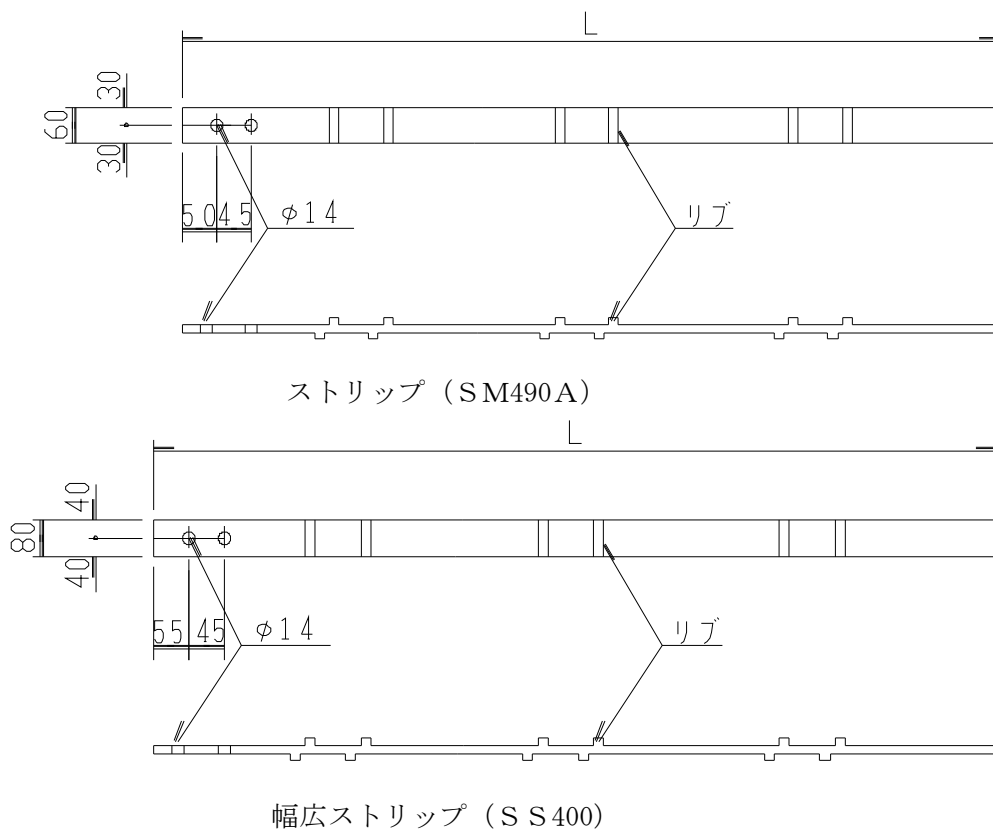
図-15 ストリップ
