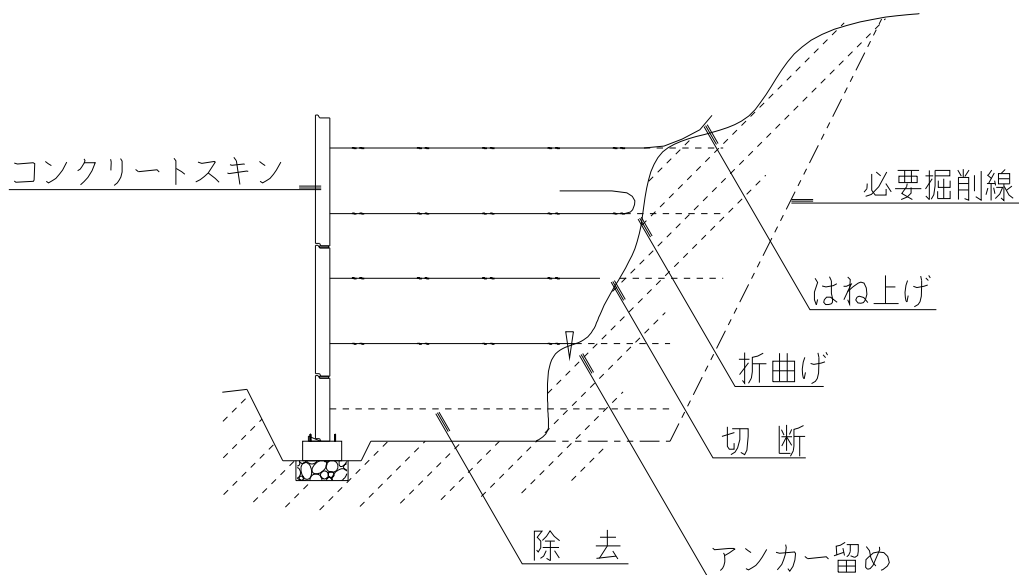
図-59 ストリップ取り付け時の禁止事項
