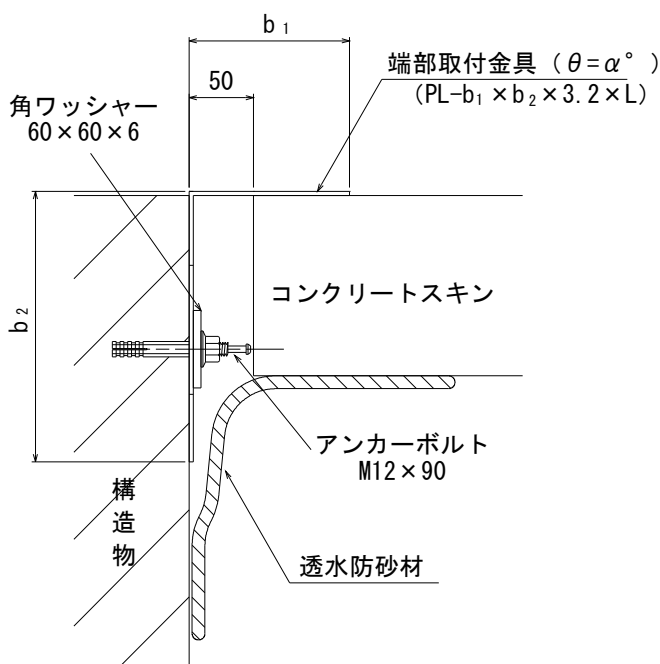
図-29 端部取付金具の設置例
