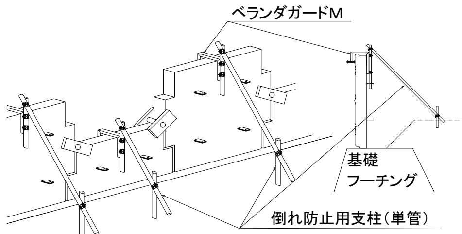
図-56 前面から指示できない場合のコンクリートスキンの転等防止策の例
