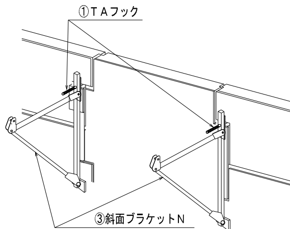
図-69 TAブラケットの取付
