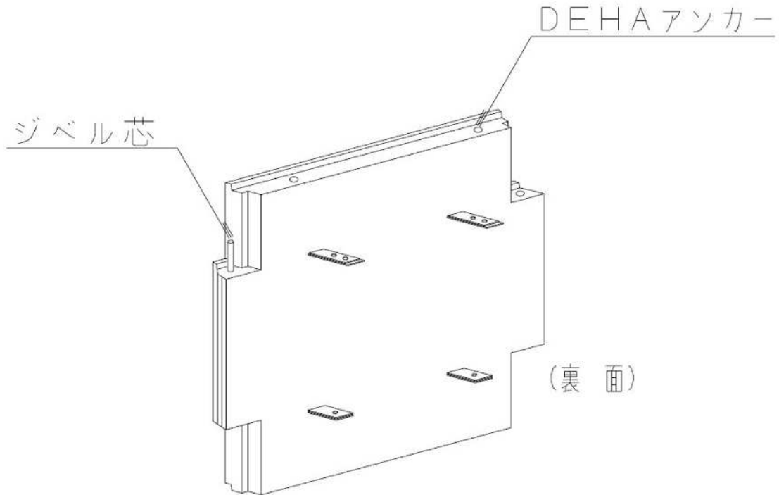
図-4 スキン構造図
