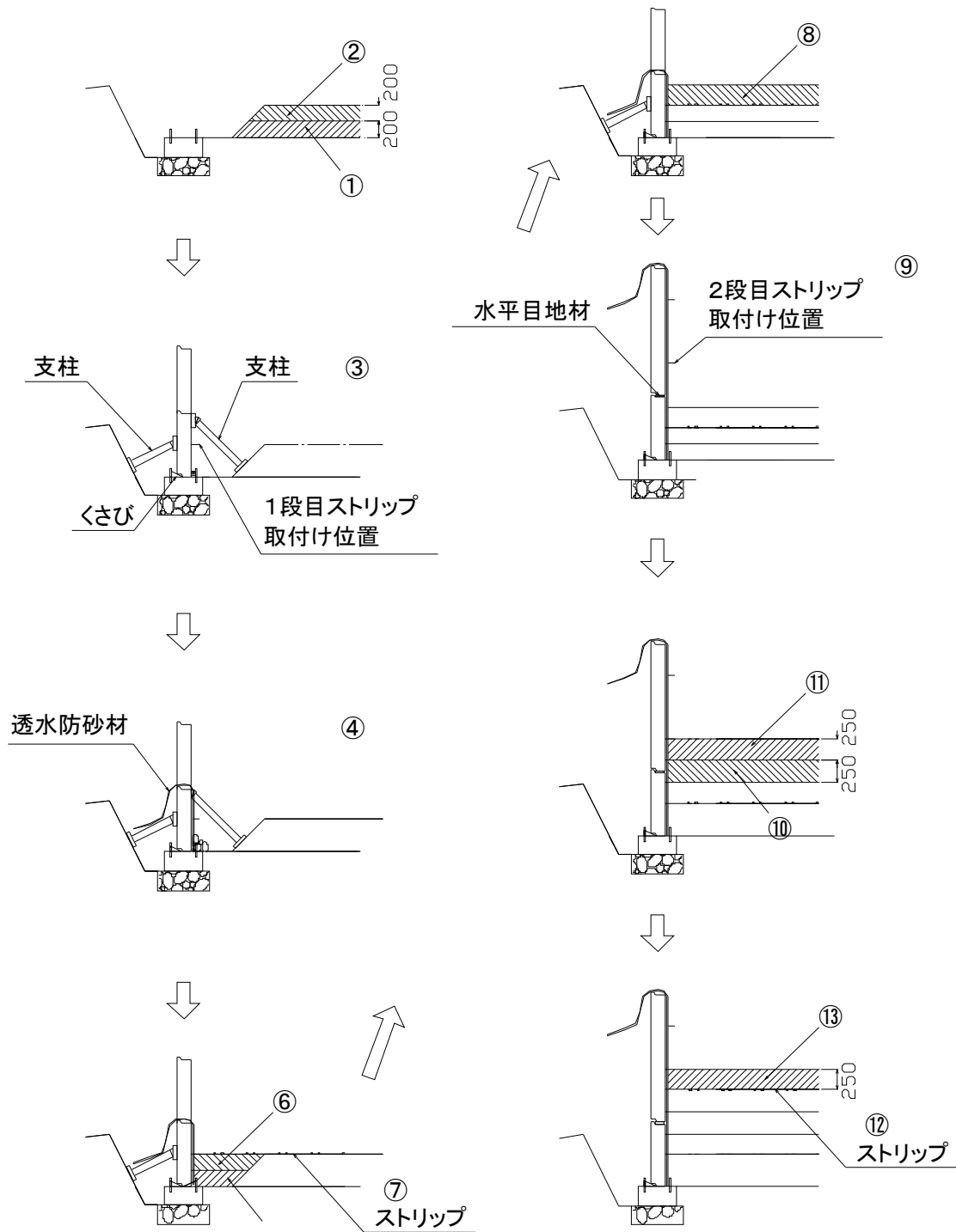
図-39 スキンパネルの組み立てから盛土工 (概略フロー)
