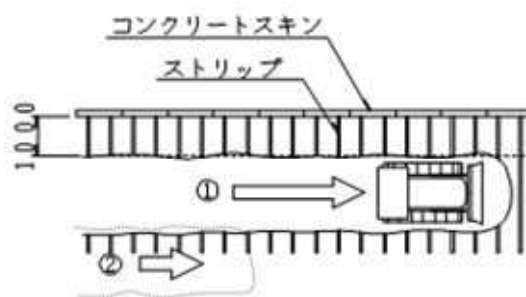
図-58 大型機械の走行
