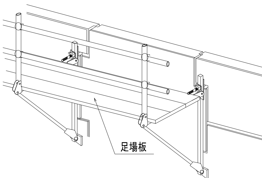
図-71 足場材の設置
