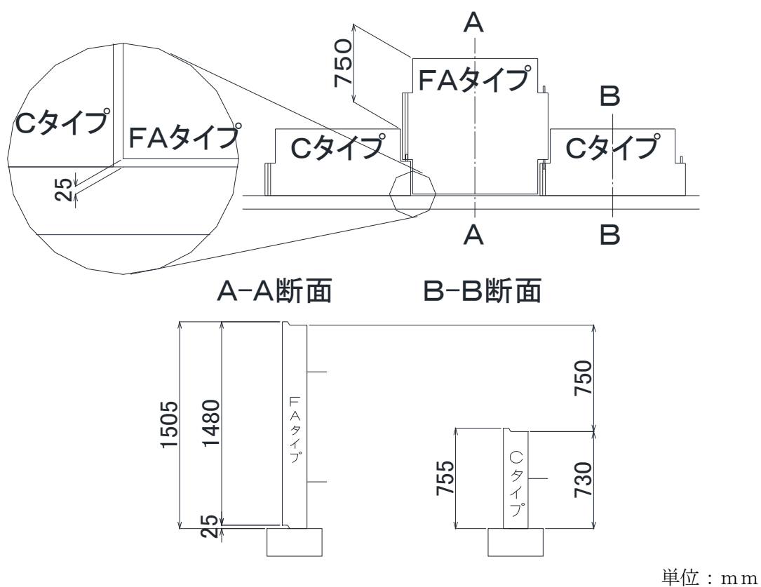
図-49 最下段スキン設置時の注意事項
