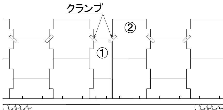
図-52 目地部のスキンの固定方法の例 (その1)
