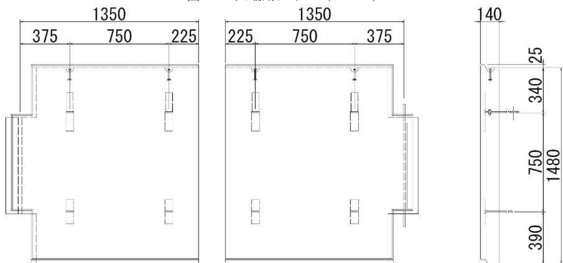
図-9 天端用タイプ (D P 2)
