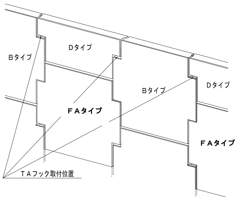
図-66 TAフックの取付け位置
