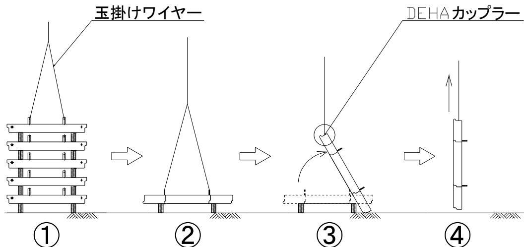
図-42 吊り上げ手順
