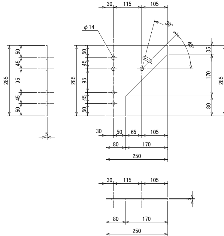
図-26 ガセットプレート
