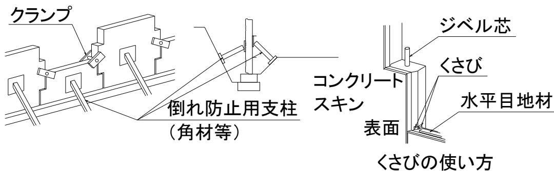
図-46 クランプ・くさびの使い方と支保工の例
