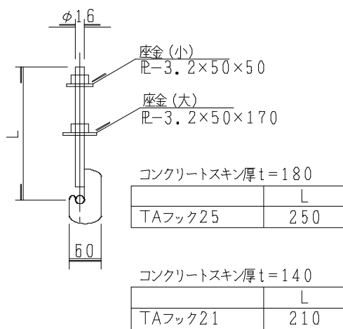
図-63 TAフック
