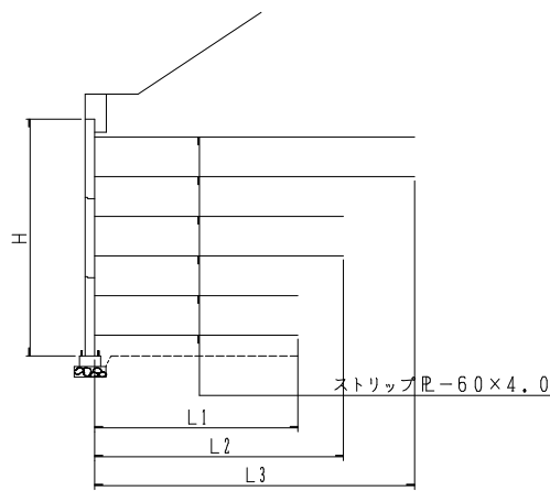
図-2 A-A横断面図 (例)
