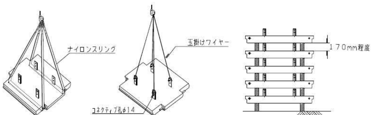
図-32 コンクリートスキン
