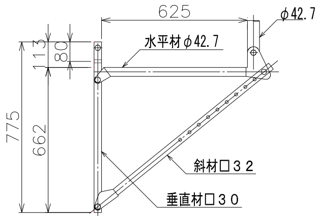
図-64 斜面ブラケットN
