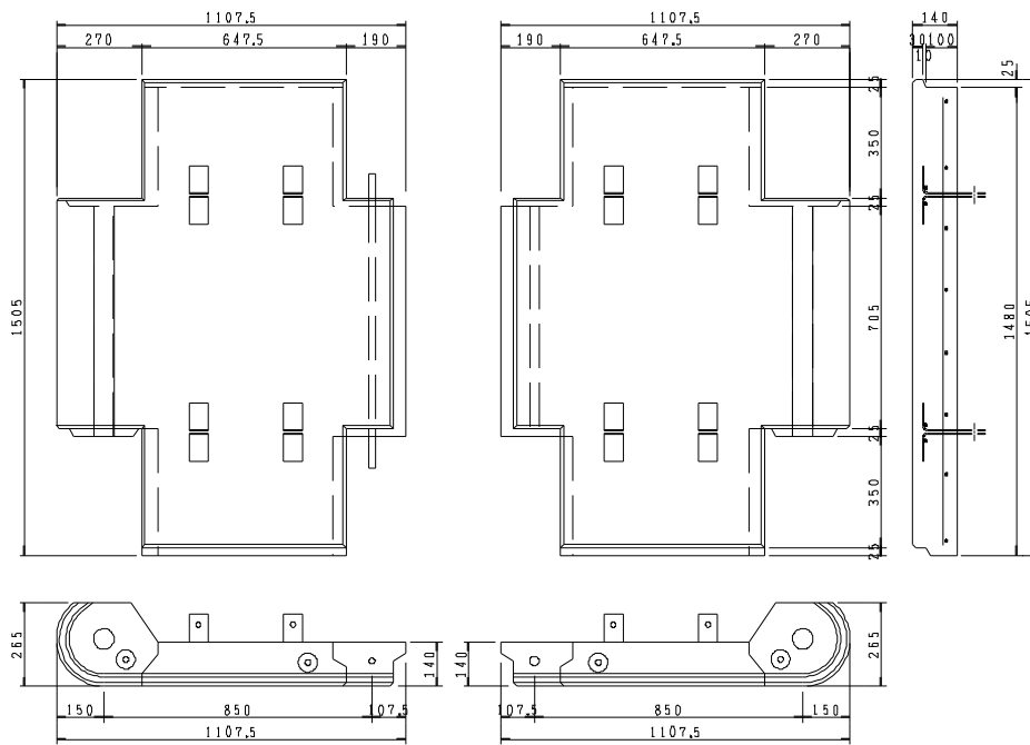
図-20 標準タイプ (MAL 4, MAR 4)
