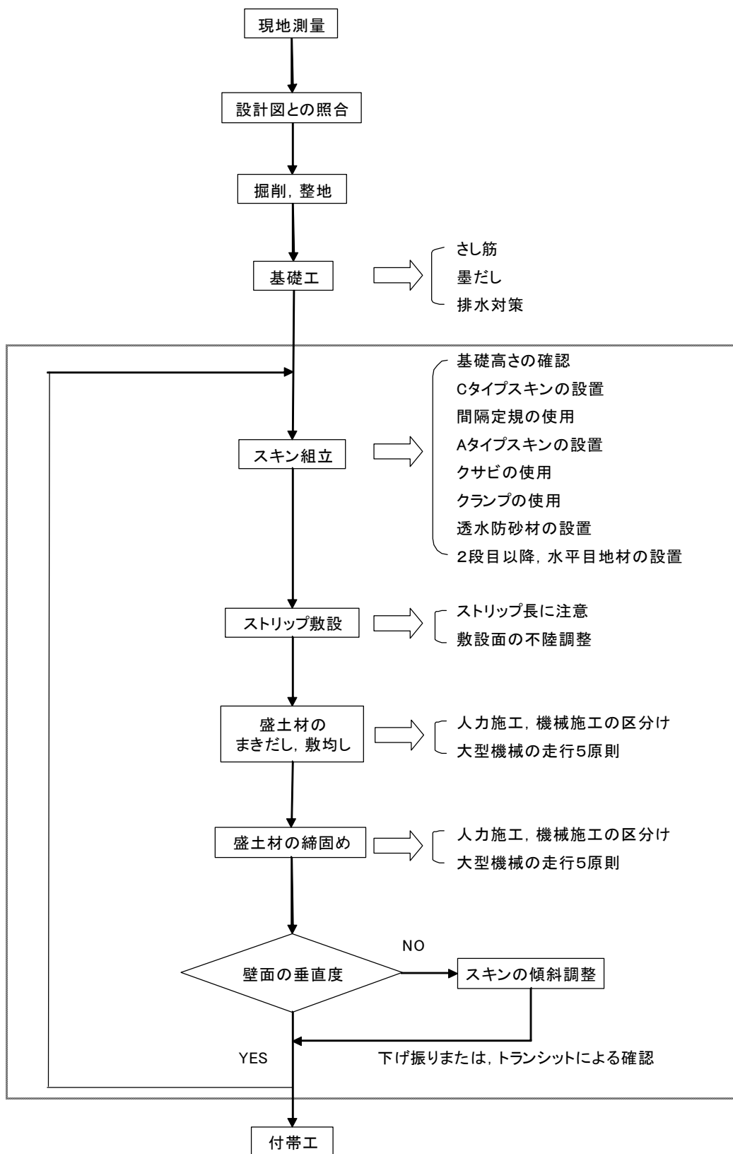
図-31 施工手順
