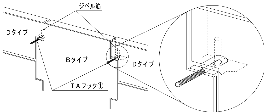
図-67 TAフック取付
