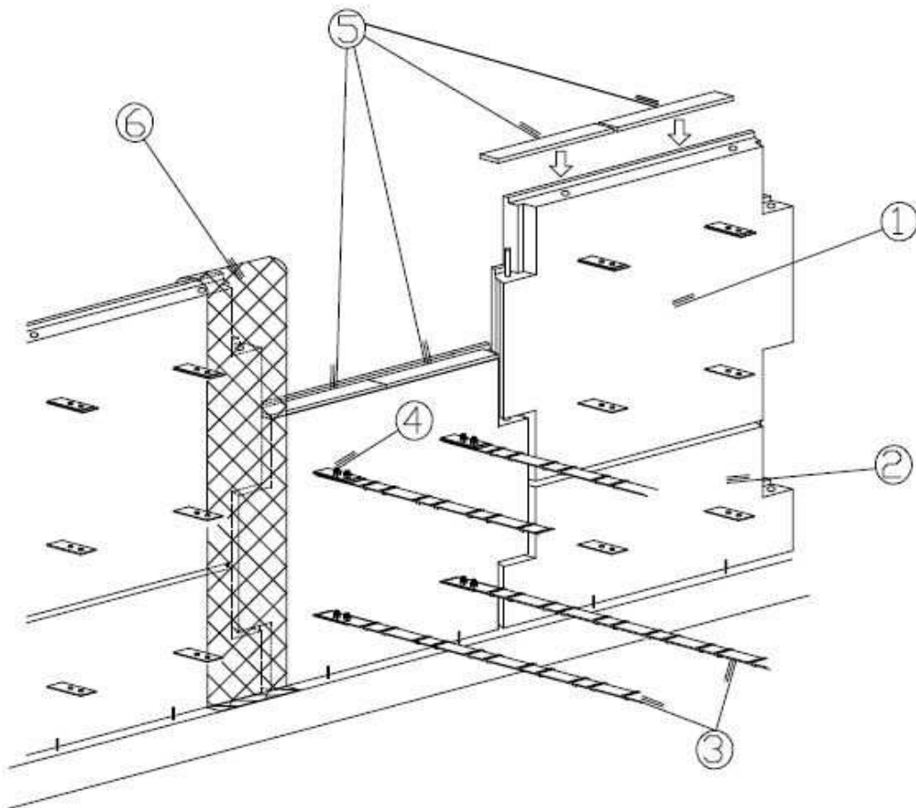
図-3 構造図(裏面)
