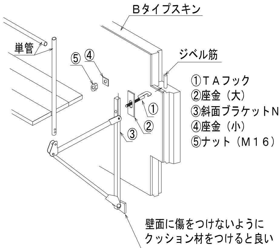
図-65 全体組立図
