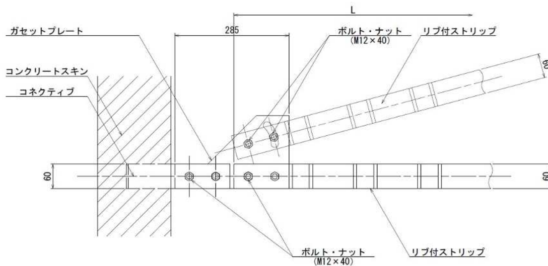
図-27 ガセットプレートの使用例
