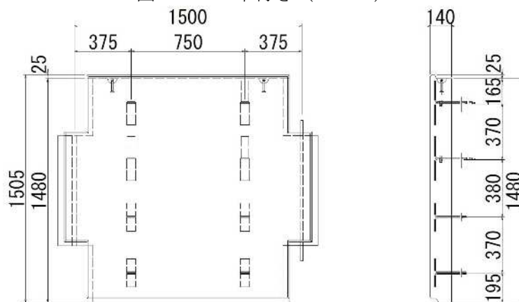
図-13 8本付き (FA8)
