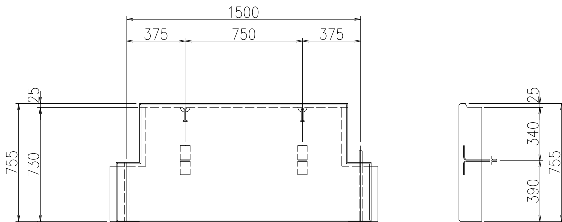
図-8 最下段用タイプ (C 2)
