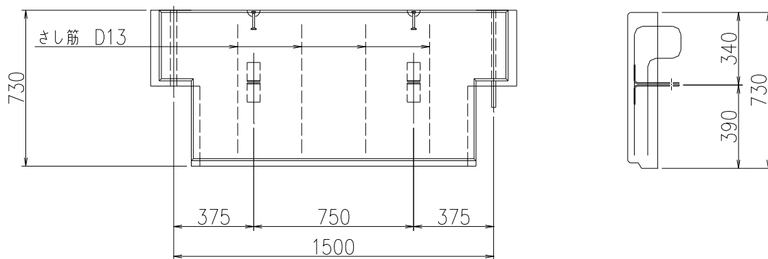
図-8 最下段用タイプ (C 2)
