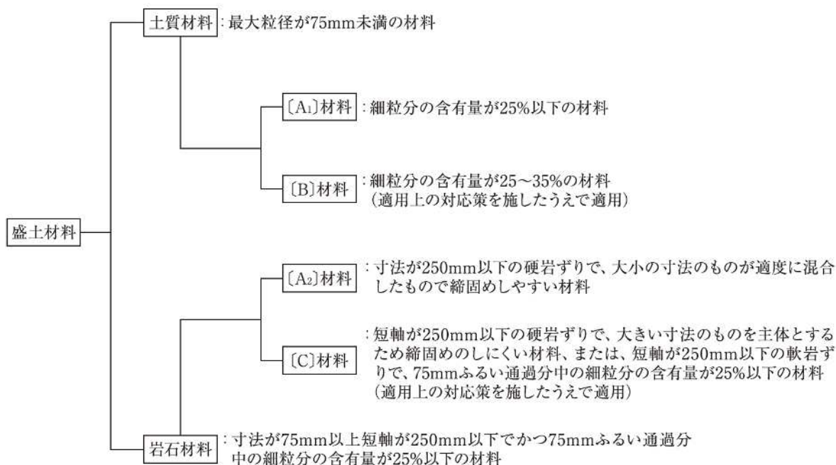
図-30 盛土材料の適用範囲
