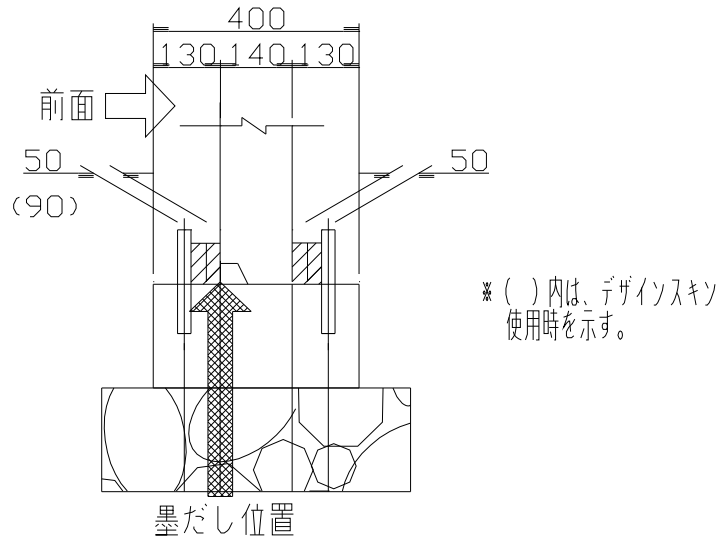
図-40 墨だし位置
