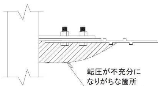
図-57 ストリップ取付図
