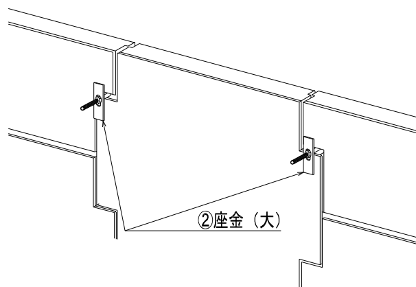
図-68 TAフックの固定
