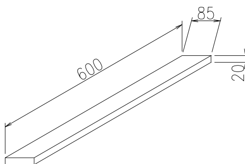
図-18 水平目地材
