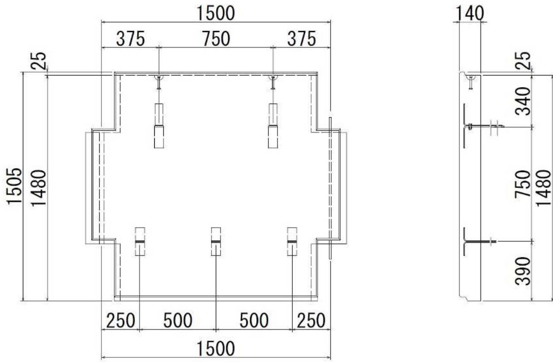
図-6 標準タイプ ( F A 5 )
