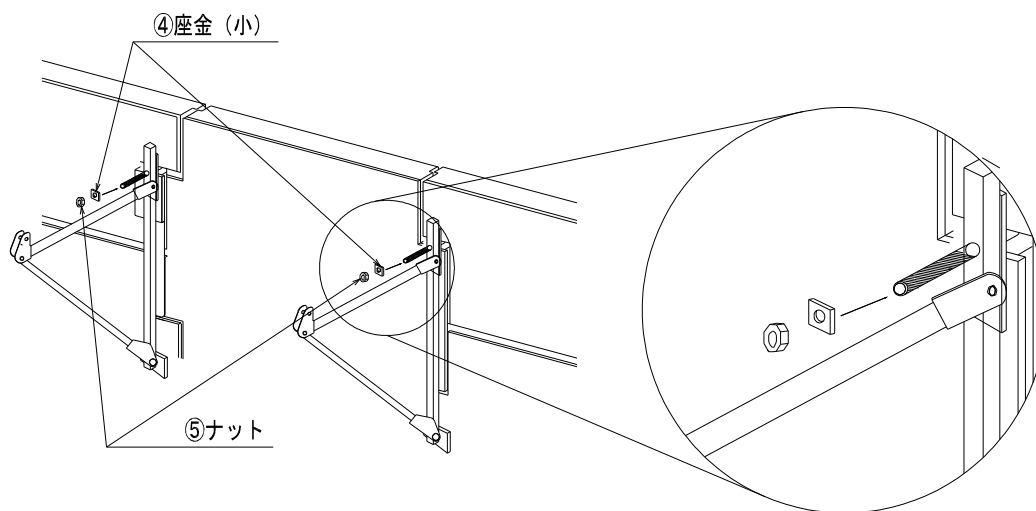
図-70 TAブラケットの固定
