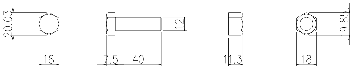
図-17 ボルト・ナット
