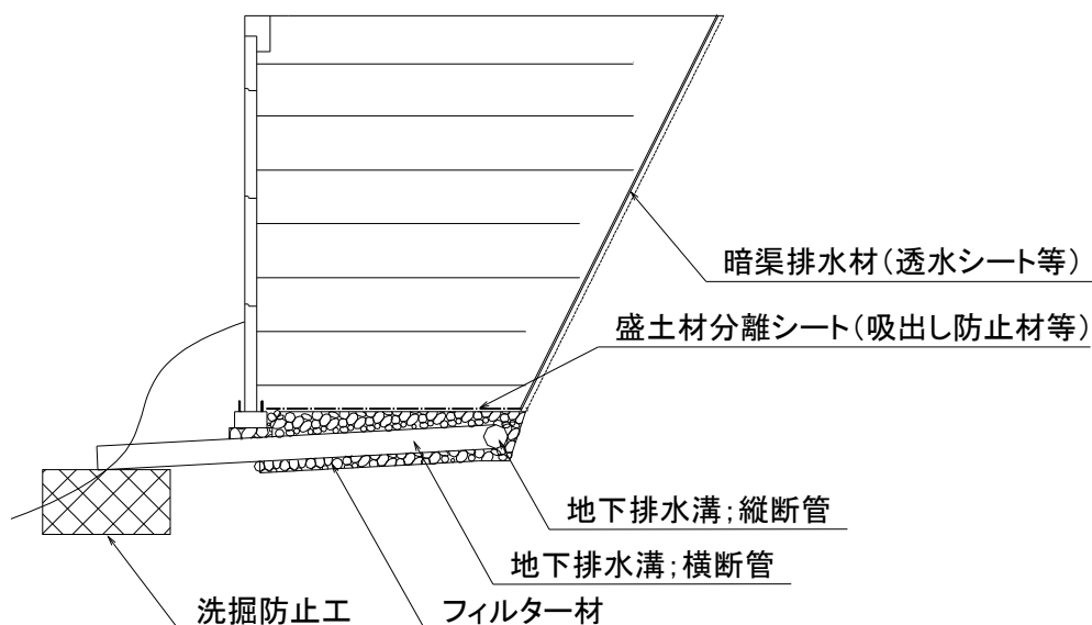
図-60 排水工例
