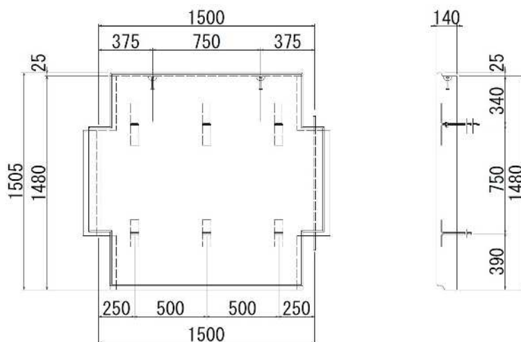
図-12 6本付き (FA6)
