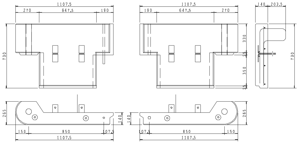
図-22 最下段用 (MCL 2, MCR 2)
